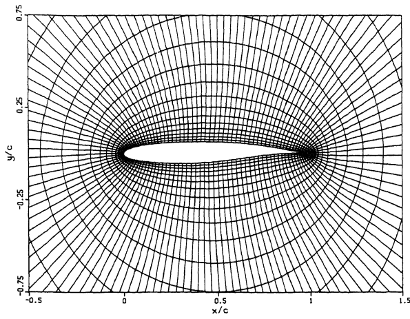
a. 128 \times 32 -grid.
