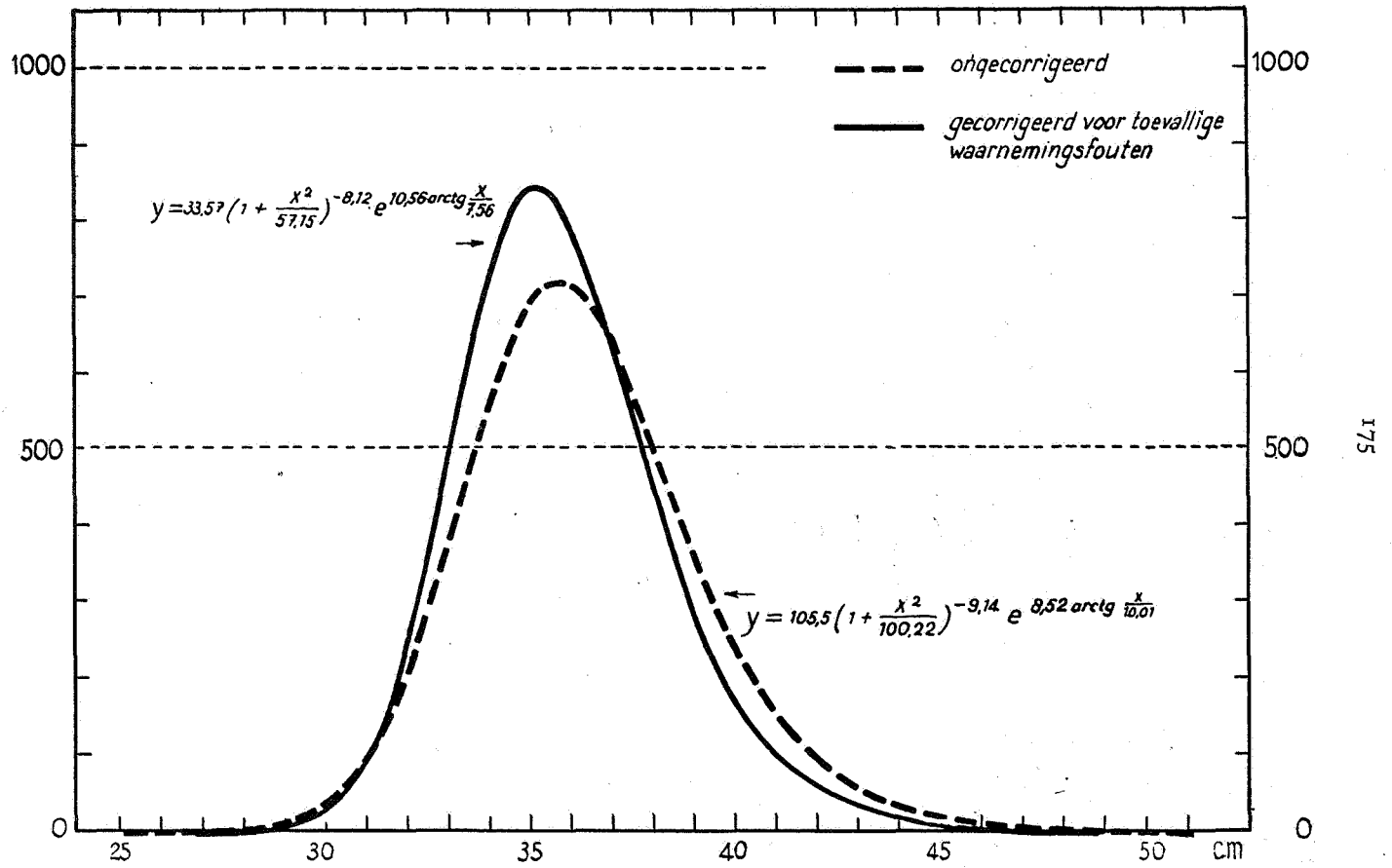
Fig. 1. Schatting van de frequentieverdeling der rugbreedte met en zonder correctie voor meetfouten.
