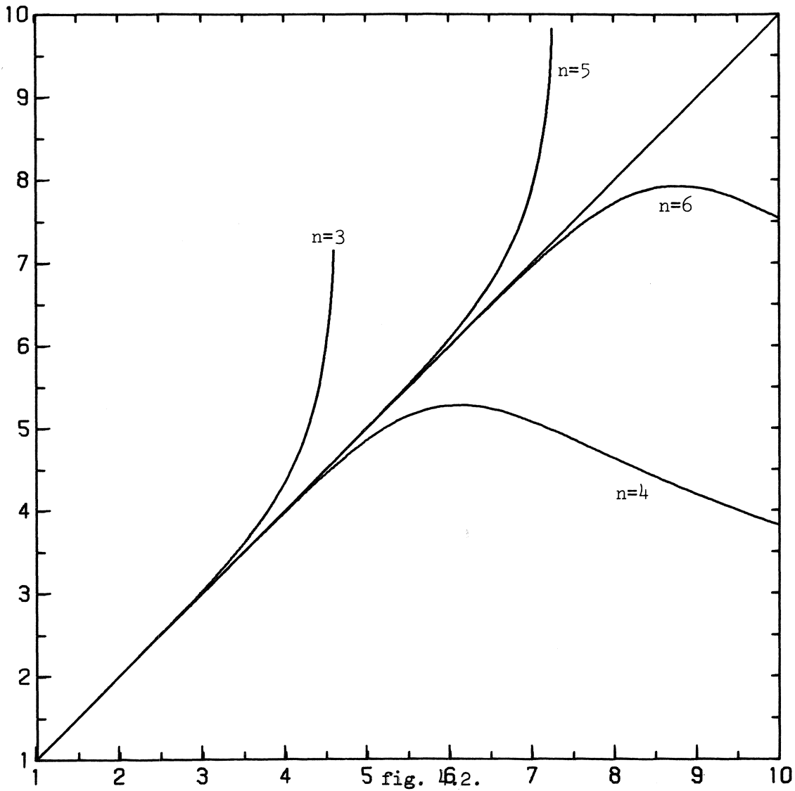
In fig. 4.2. zijn de grafieken y = x en y = \ln(E(n,n;z)) getekend voor n = 3, 4, 5, 6 . E(3,3;z) en E(5,5;z) hebben elk een pool bij 4,6 resp. 7,3. K_{n+\frac{1}{2}}(-z) heeft nl. één reëel nulpunt voor oneven n en geen reëel nulpunt voor even n .
