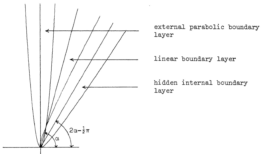
Fig. 1 \alpha < \frac{1}{2}\pi
