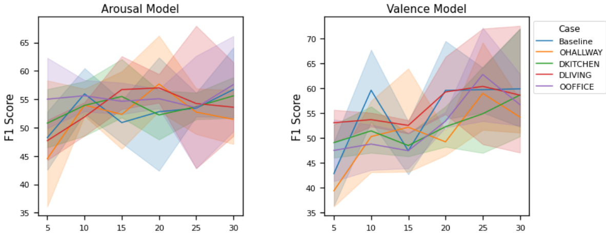
Figure 6.9: K-EmoCon : Summary of Query Set F1 score ( F1 ) for different cases
