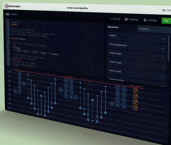
Figuur 1: De programmeeromgeving van Quantum Inspire toont de qubits op de horizontale lijnen en de bewerkingen als verticale lijntjes met bolletjes die aangeven welke qubits met elkaar wisselwerken. Een vierkantje met een letter erin is een operatie op één enkele qubit. De X-operatie is een bitflip (0 wordt 1 en 1 wordt 0), de H (= Hadamard) operatie brengt een qubit in een quantumsuperpositie van 0 en 1. Het +-teken is een operatie op drie qubits (flip de qubit indien de twee qubits waarmee het plusje verbonden is beide de waarde 1 hebben). Credits: QuTech.
