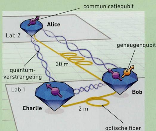
Figuur 2: Drie knooppunten, genaamd Alice, Bob en Charlie, bevinden zich in twee afzonderlijke laboratoria op de Delftse campus. Elk knooppunt bevat een communicatiequbit (paars) gebaseerd op een roosterdefect in een diamantje. Bij Bob wordt bovendien een kernspinqubit (oranje) gebruikt als geheugen. Optische fiberverbindingen tussen de knooppunten maken het mogelijk om quantumverstrengeling te genereren tussen alle drie de knooppunten (kronkelende lijnen). Figuur aangepast uit [7].
