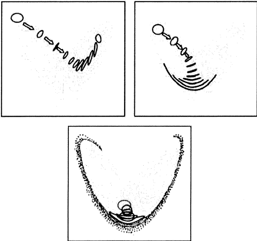
Figuur 1. Ensemble simulaties van het systeem Lorenz (1963) met verschillende graden van voorspelbaarheid. (Bron: Tim Palmer, ECMWF.)
