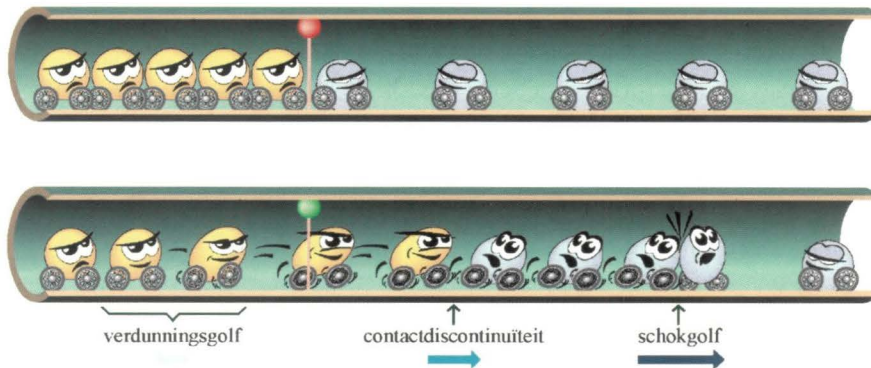
Figuur 11: 'Schokbuis'. Boven : rusttoestand met in linker en rechter gedeelte: hoge respectievelijk lage druk en dichtheid. Onder : bewegingstoestand met naar rechts lopende schokgolf en contactdiscontinuïteit en naar links lopende verduunningsgolf. (tekening: Tobias Baanders).
