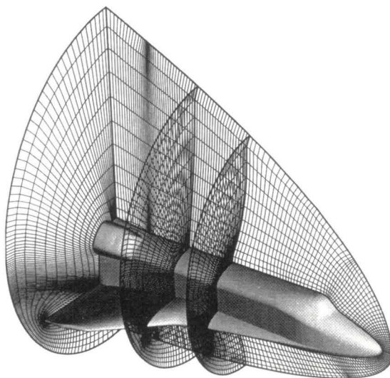
Figuur 15: Doorsneden van een uit zesvlakjes opgebouwd rooster om de Space Shuttle.
