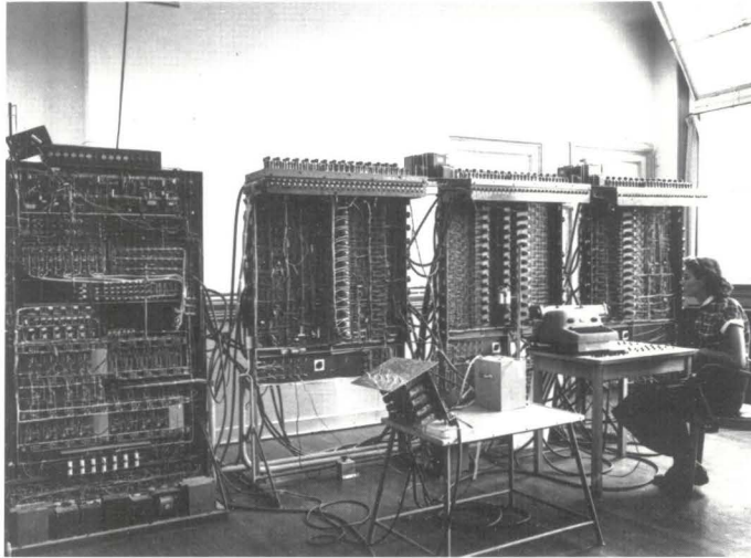
Figuur 8: De eerste computer bij het CWI en in Nederland, de ARR A I in zijn uiteindelijke opstelling. Van links naar rechts: voedingsframe en de drie aritmetische registers. Op het tafeltje in het midden staat de ponsbandlezer. De ongeveer 1200 relais zitten aan de achterkant van de machine.
