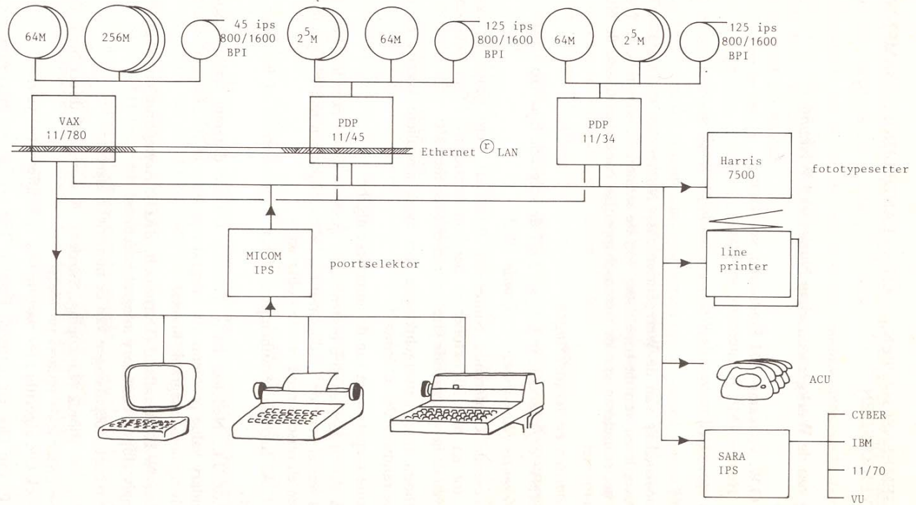
Schema : Computerapparatuur
