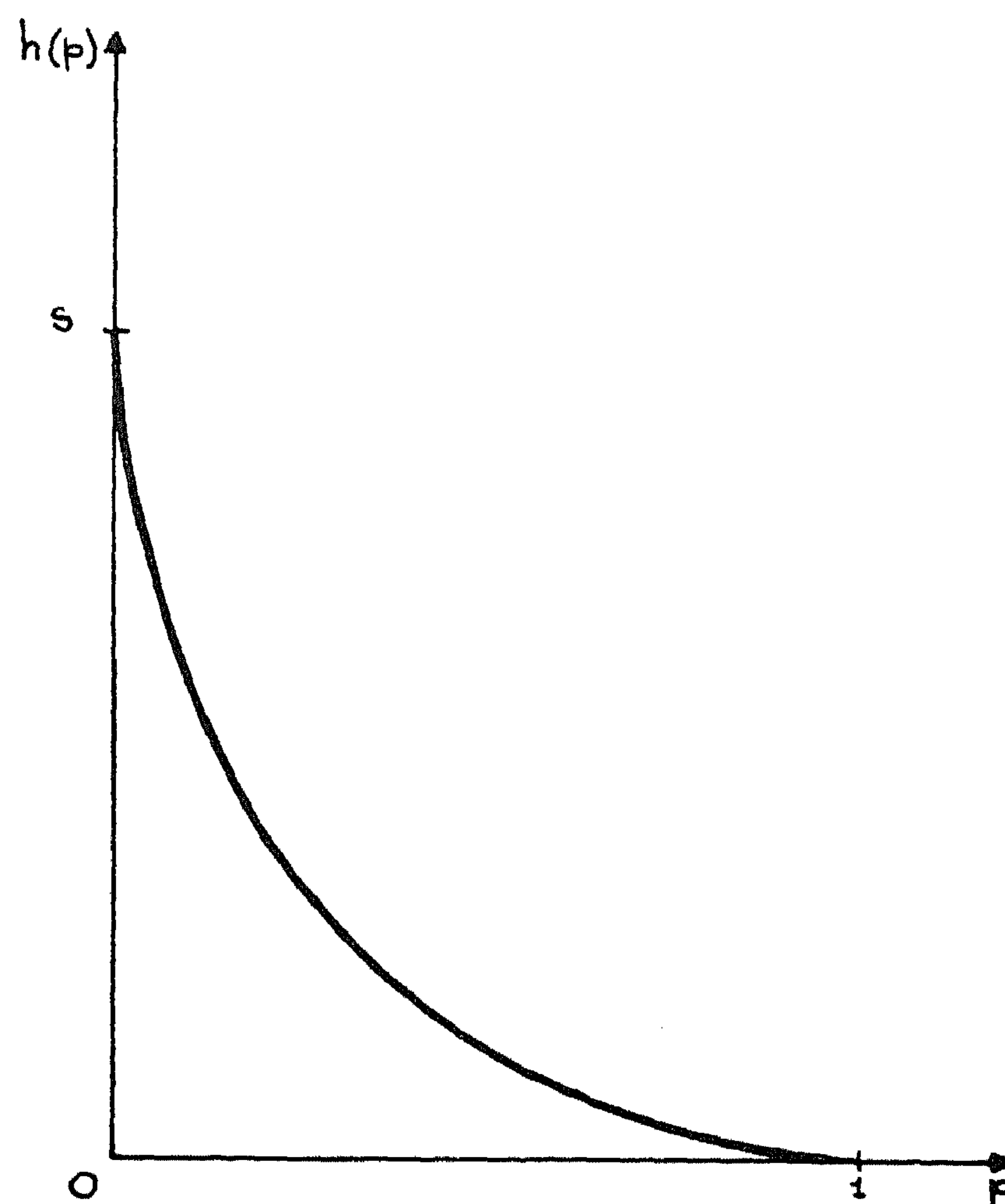
Fig. 4.1. j -vormige a priori-verdeling van \underline{p} .
