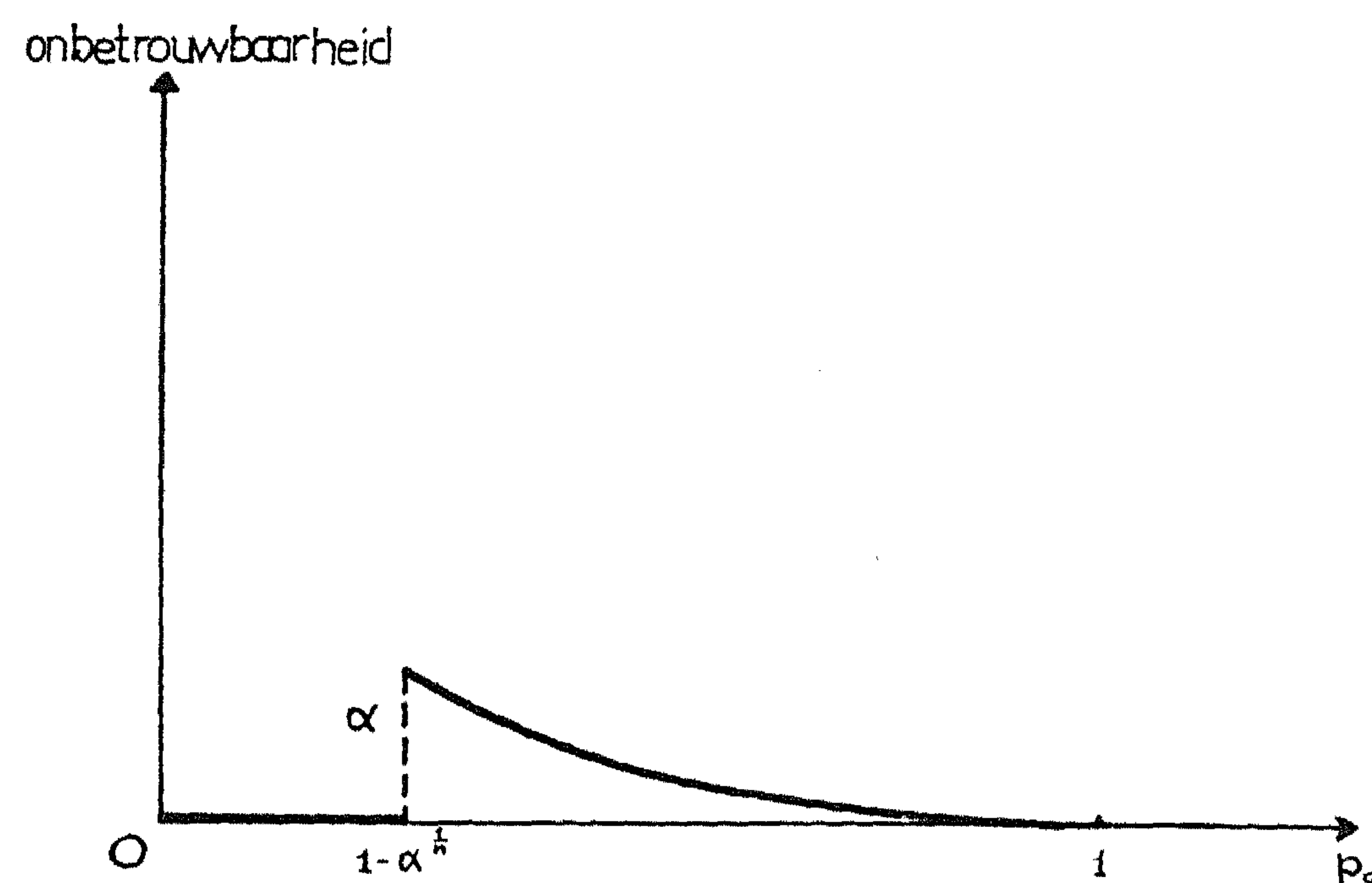
Fig. 3.1. Onbetrouwbaarheid bij de gewijzigde interpretatie van de methode van De Wolff.
