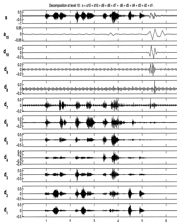
FIGUUR 11. Decompositie van het spraaksignaal "Ik zie ..."
