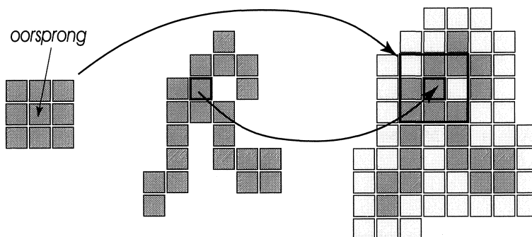
FIGUUR 5. Van links naar rechts: het structurend element A , de input verzameling X (donkere pixels) en de gedilateerde X \oplus A (lichte en donkere pixels).
