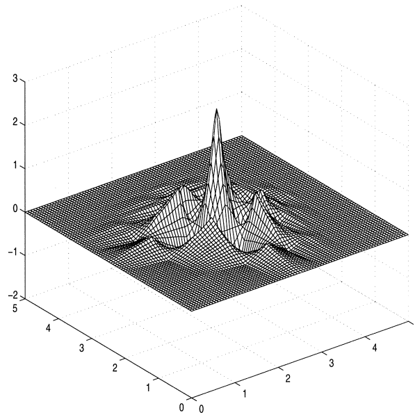
FIGUUR 9. Een bivariate Daubechies wavelet, orde 3 en diagonale detail
