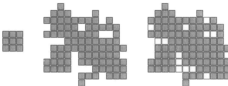
FIGUUR 10. Van links naar rechts: het structurerend element A , de input verzameling X en de sluiting X \bullet A .
