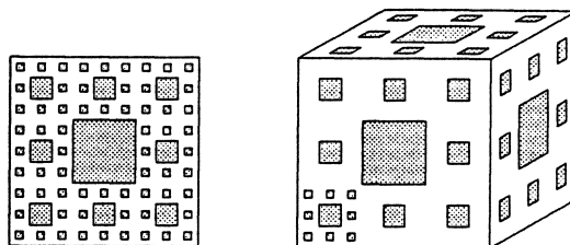
FIGUUR 4. Vloerkeed van Sierpiński (links) en Spons van Menger (rechts)
