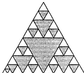
FIGUUR 3. De Sierpiński-kromme
