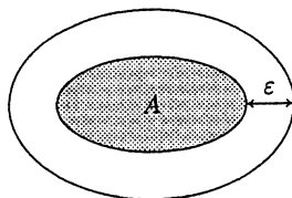
FIGUUR 7. B_\epsilon(A)
