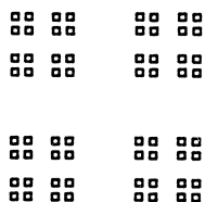
FIGUUR 5. C \times C
