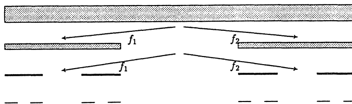
FIGUUR 1. Het Cantor-discontinuum
