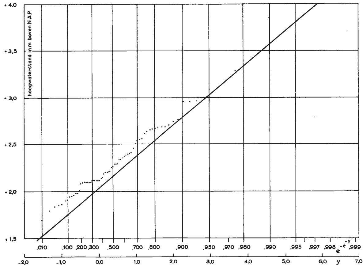
Figuur 7.7. De verdeling van de jaarmaxima der hoogwaterstanden uit de jaren 1888 tot en met 1956 en een daarmee vergelijkbare verdelingsfunctie, op grond van de baanselectiewaarnemingen
