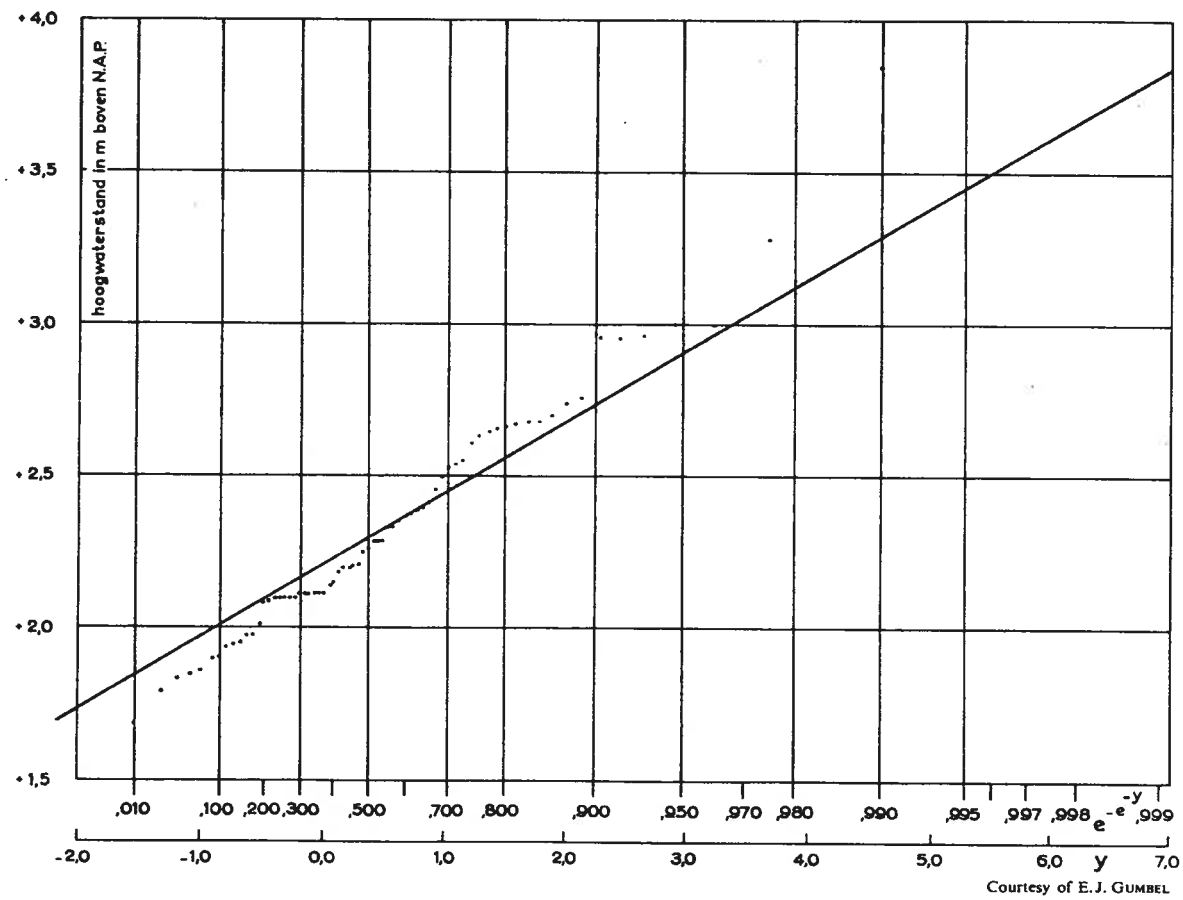
Figuur 7.6. De verdeling van de jaarmaxima der hoogwaterstanden uit de jaren 1888 tot en met 1956 en een daarmee vergelijkbare verdelingsfunctie, op grond van alle waarnemingen
