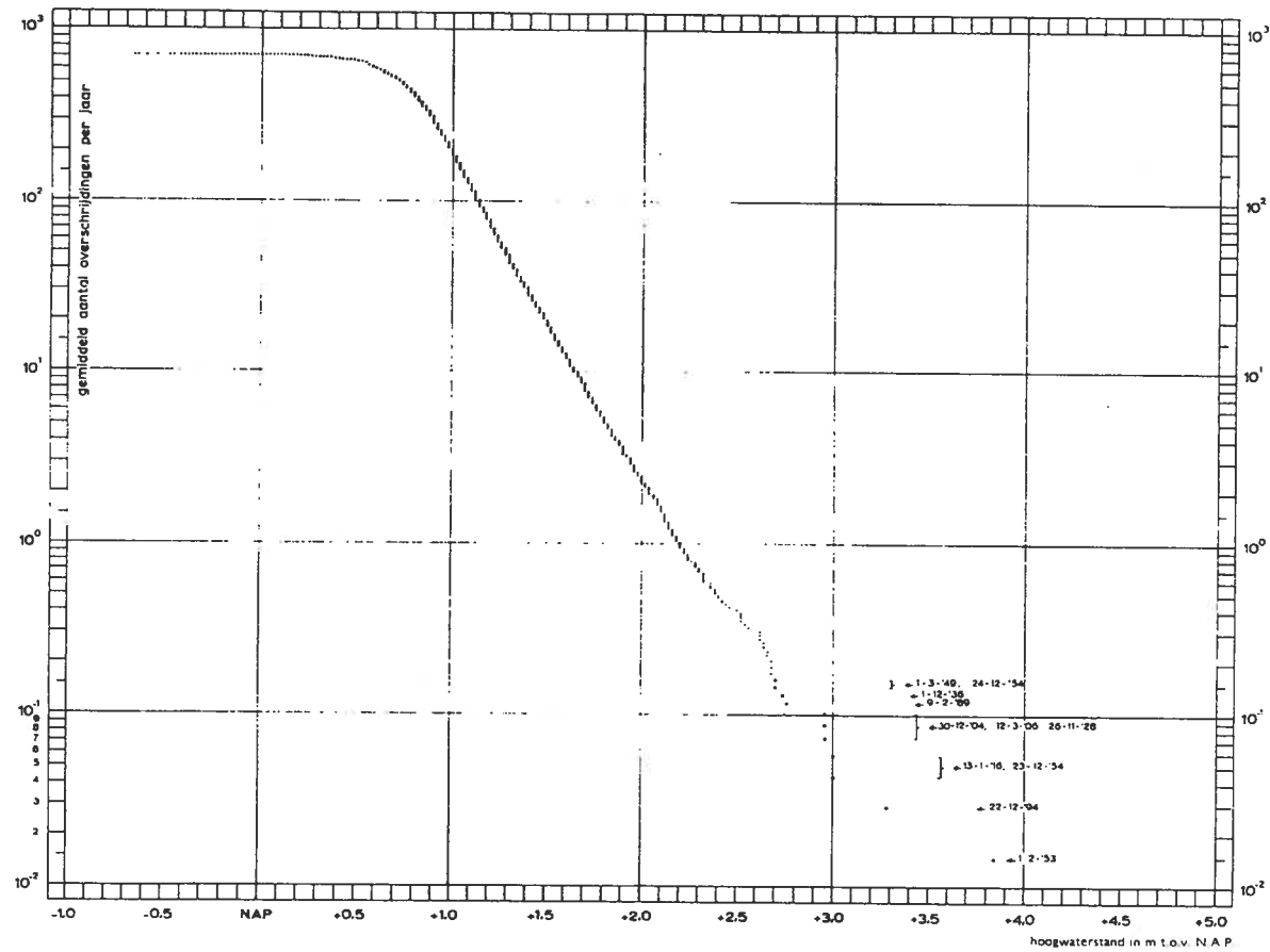
Figuur 7.1. Het gemiddeld aantal overschrijdingen per jaar van het peil h, afkomstig van alle hoogwaterstanden uit de jaren 1888 tot en met 1956
