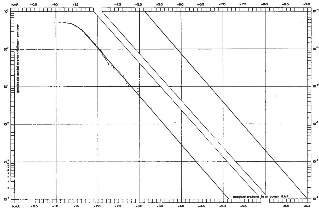
Figuur 7.5. Het gemiddeld aantal overschrijdingen per jaar van het peil h , afkomstig van de hoogste hoogwaterstanden der naar banen geselecteerde depressies, uit de maanden januari, november en december der winters 1888/'89 tot en met 1938/'39 en 1945/'46 tot en met 1956/'57, met een daaraan aangepaste rechte
