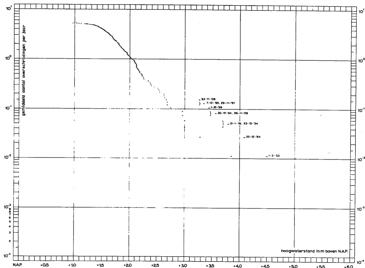
Figuur 7.3. Het gemiddeld aantal overschrijdingen per jaar van het peil h, afkomstig van de hoogste hoogwaterstanden der naar banen geselecteerde depressies, uit de maanden januari, november en december der winters 1888/'89 tot en met 1938/'39 en 1945/'46 tot en met 1956/'57
